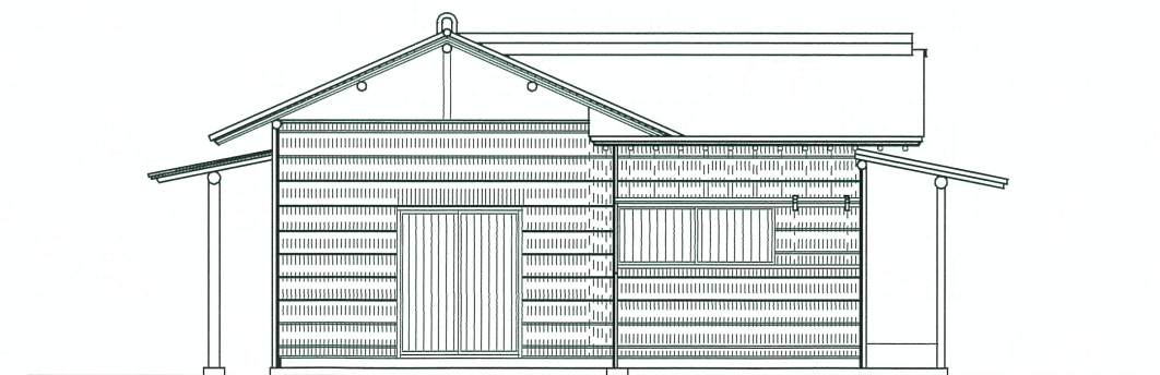
西側立面図
