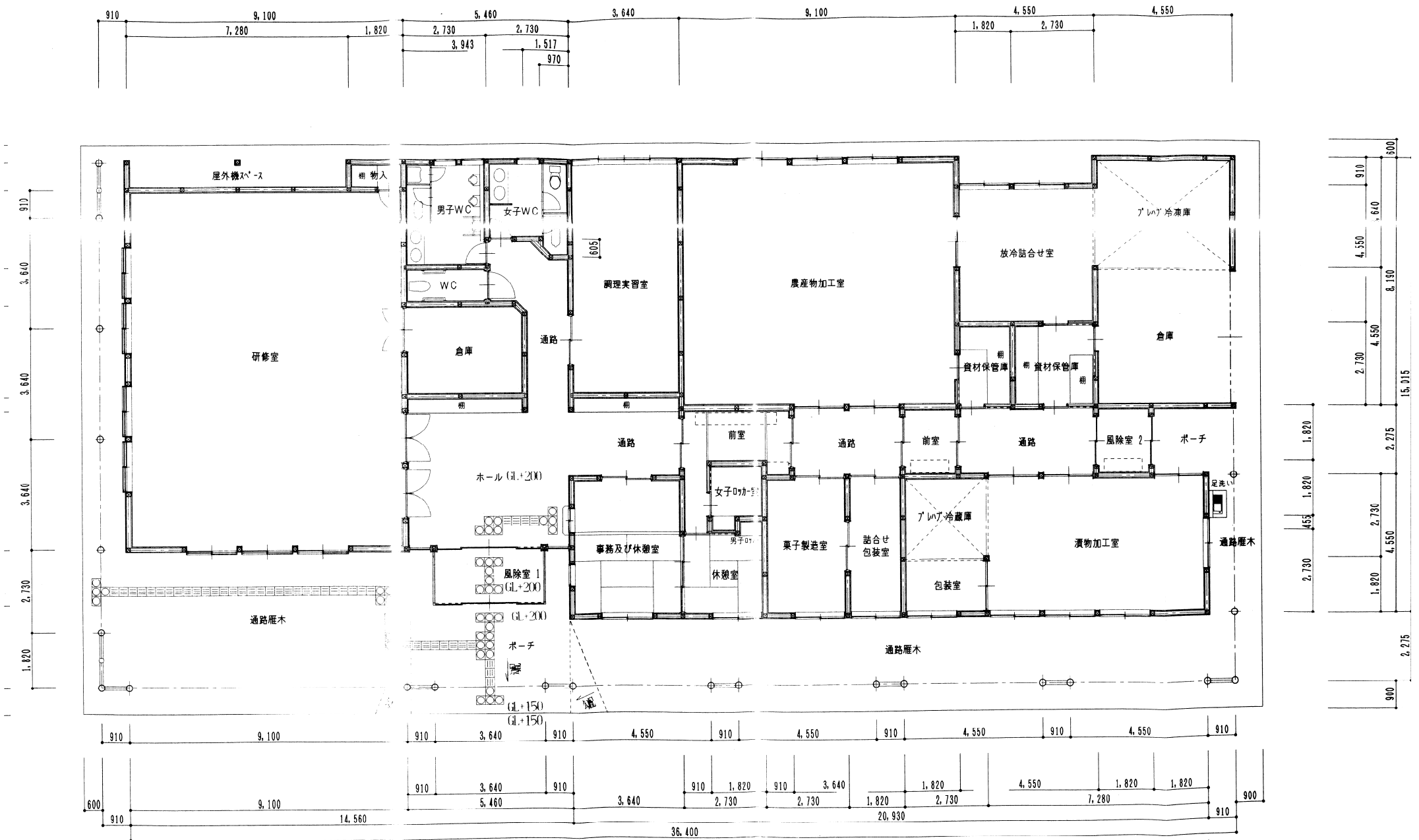
由利本荘市鳥海農産物加工施設 平面図
