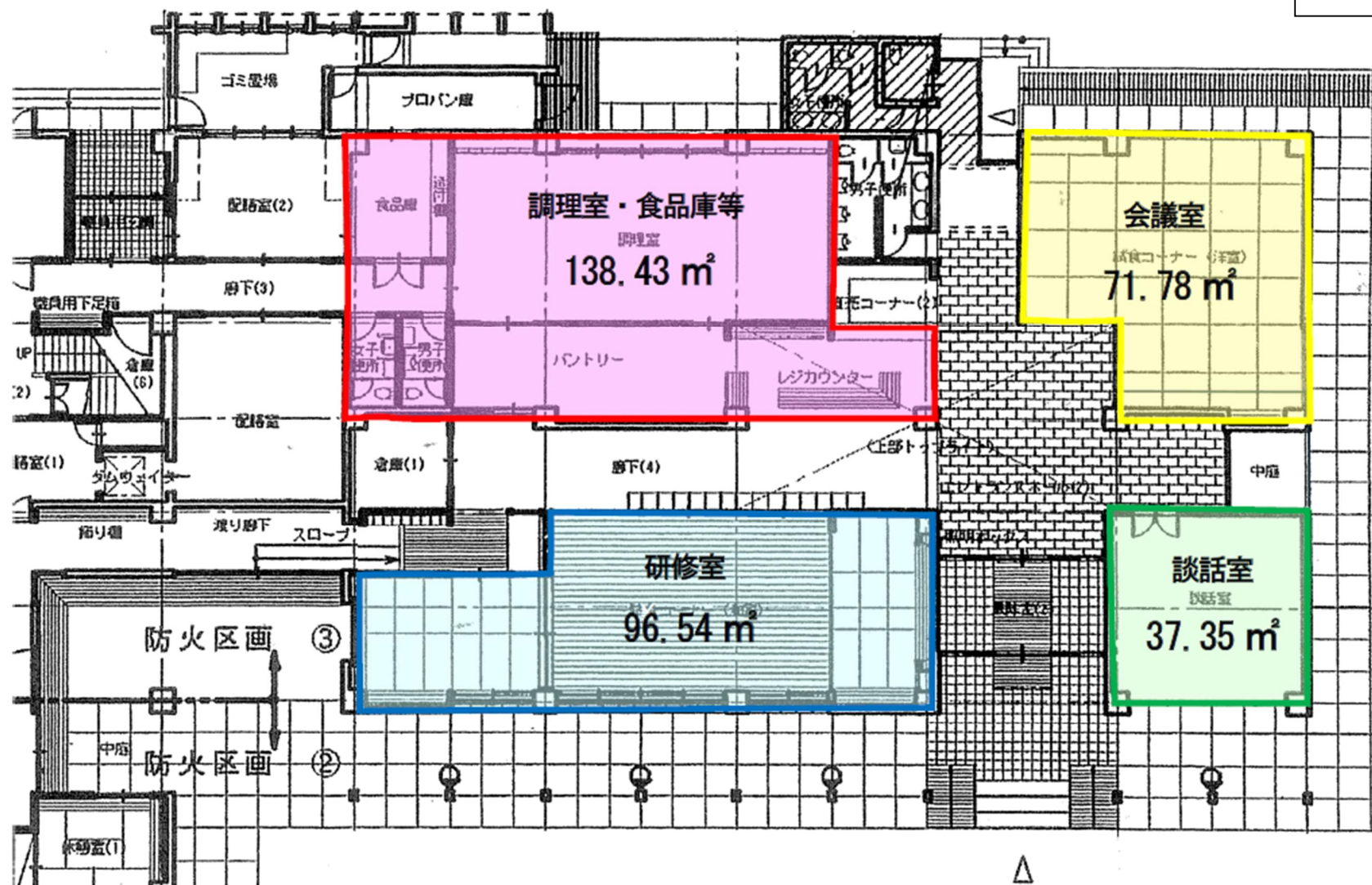
由利本荘市東由利産地形成促進施設 レストラン「やしお」 平面図
