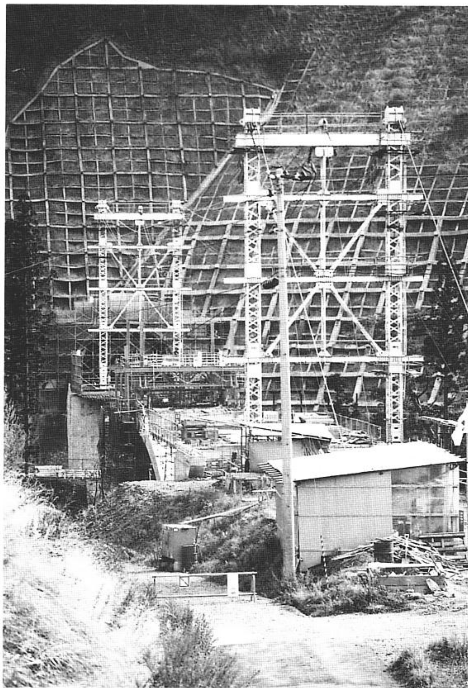
▲奥名免橋完成にむけて工事が進む国道107号
