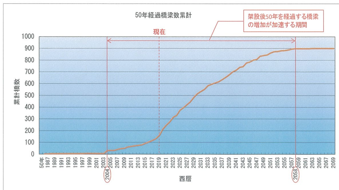
図4.2 50年経過橋梁数累計
