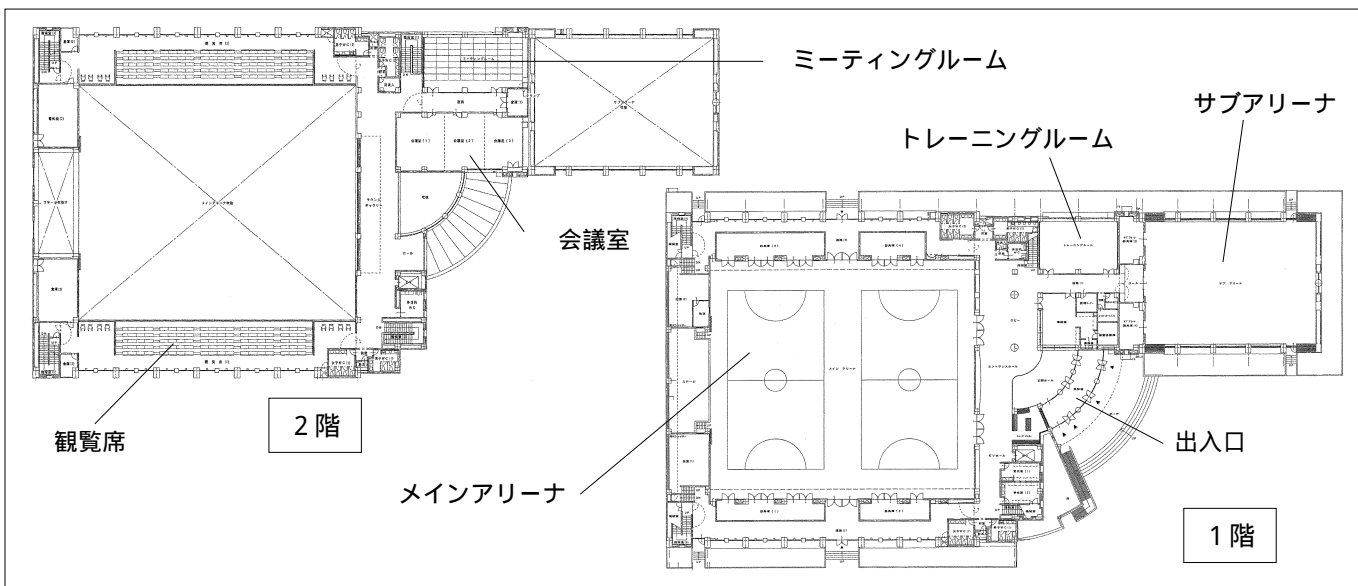
平面図
