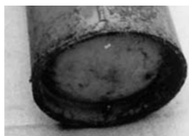
腐食した溶接部
