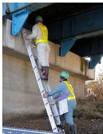
写真3.2 梯子による点検
