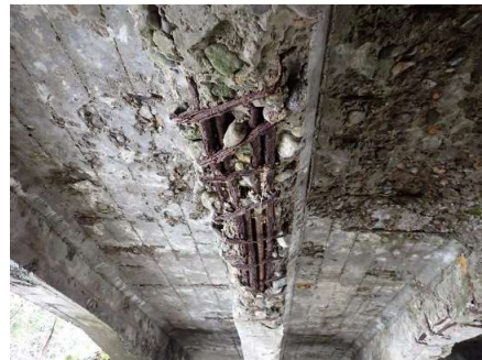
主桁の剥離・鉄筋露出
