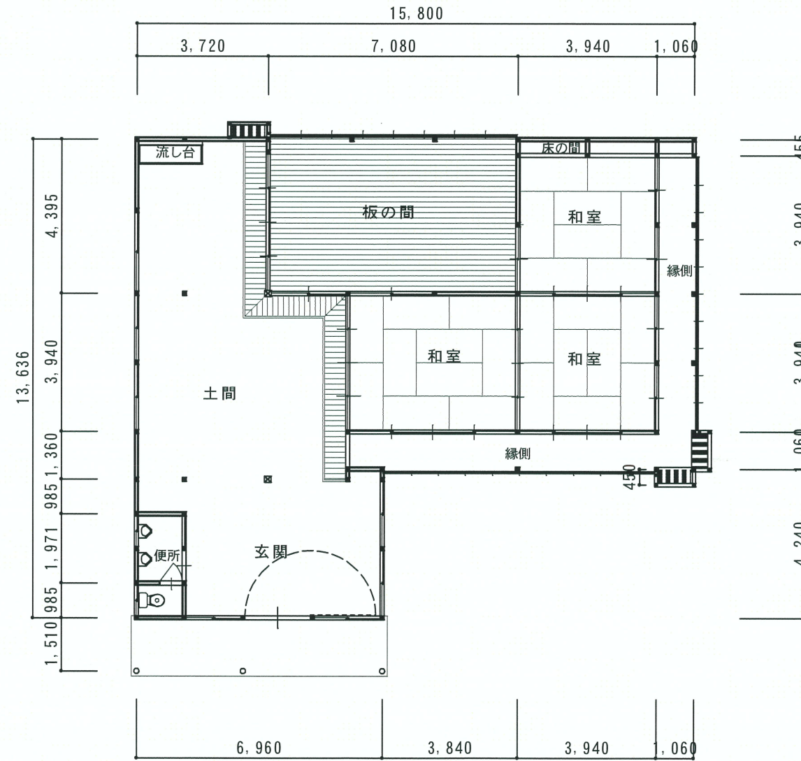
平面図 1 / 150
