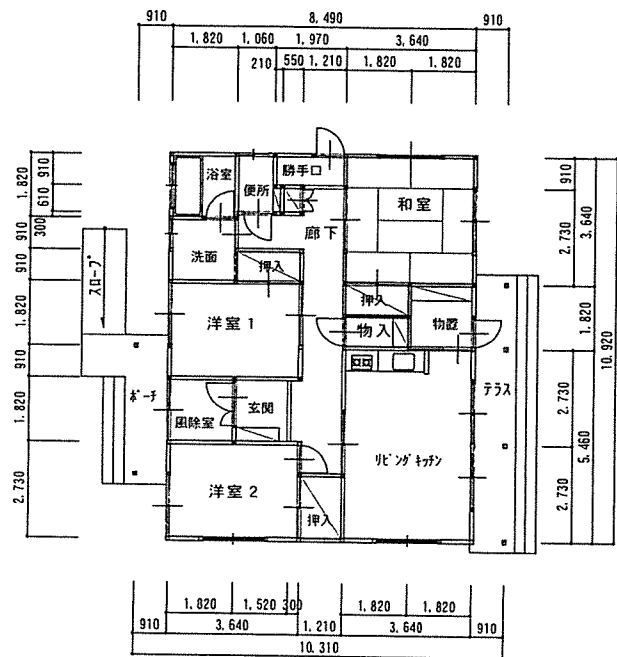
平面图 1 / 150
